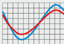
Rys.3 Prąd i napięcie na wejściu AFE współczynnik cosφ~1
