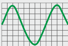
Rys.2 Czysta Moc układy AFE zwracają do sieci energię sinusoidalną – THDi <4%
